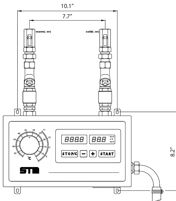
DOMIX 35
