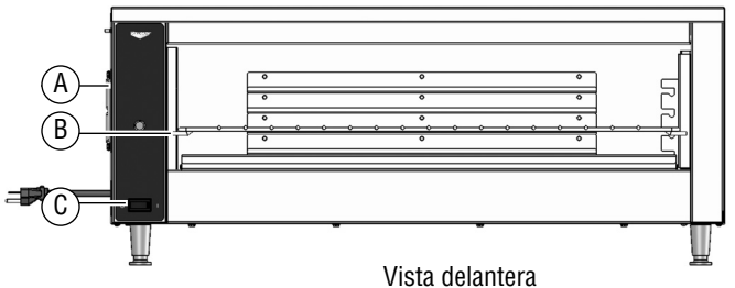
Vista delantera
