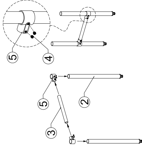
Step1
