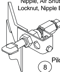
8706 (NAT) or 8707 (LP) Pilot Burner TS11K
