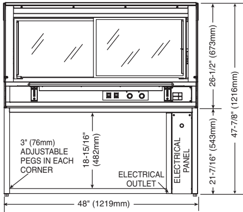
ED2SYS-48/2S
