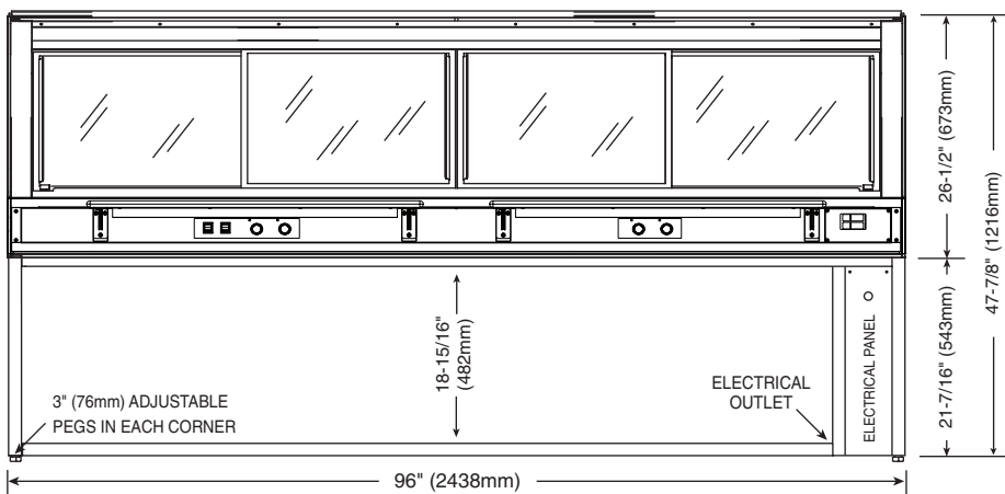
ED2SYS-96/2S
