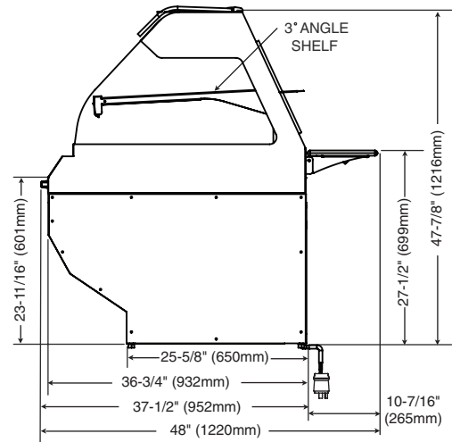
ED2SYS-2S PROFILE
